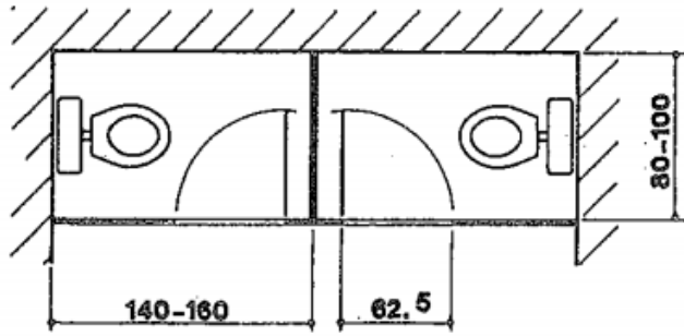
Kabinen querliegend
